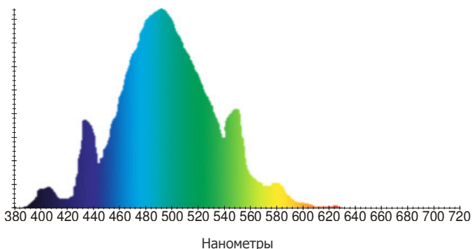
Разряд с ртутными парами при низком давлении
