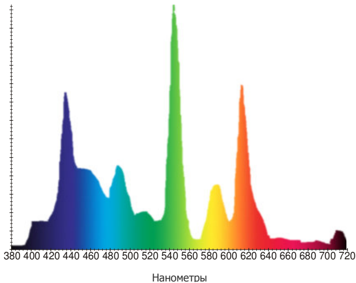
Спектральное распределение
