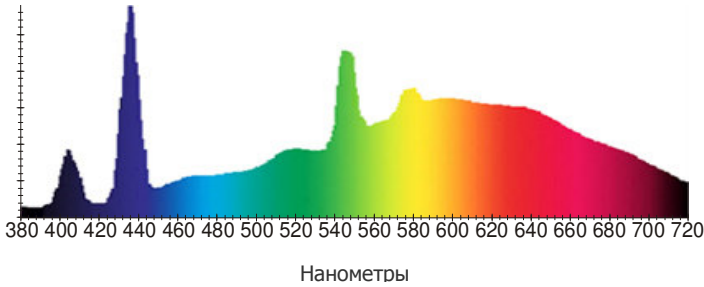
Разряд с ртутными парами при низком давлении
