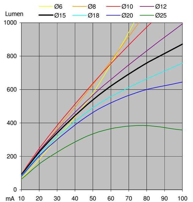
Световой поток 1 м - диам. 15 мм
