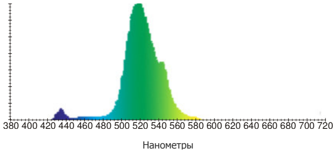
Разряд с ртутными парами при низком давлении
