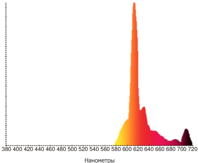
Разряд с ртутными парами при низком давлении
