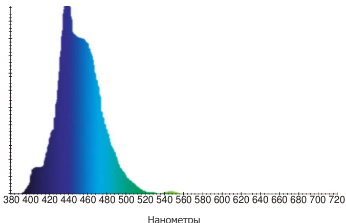
Спектральное распределение
