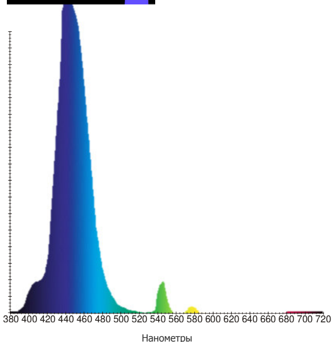
Разряд с ртутными парами при низком давлении
